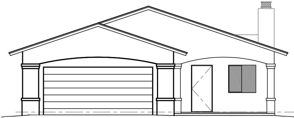
ELEVATION - A
